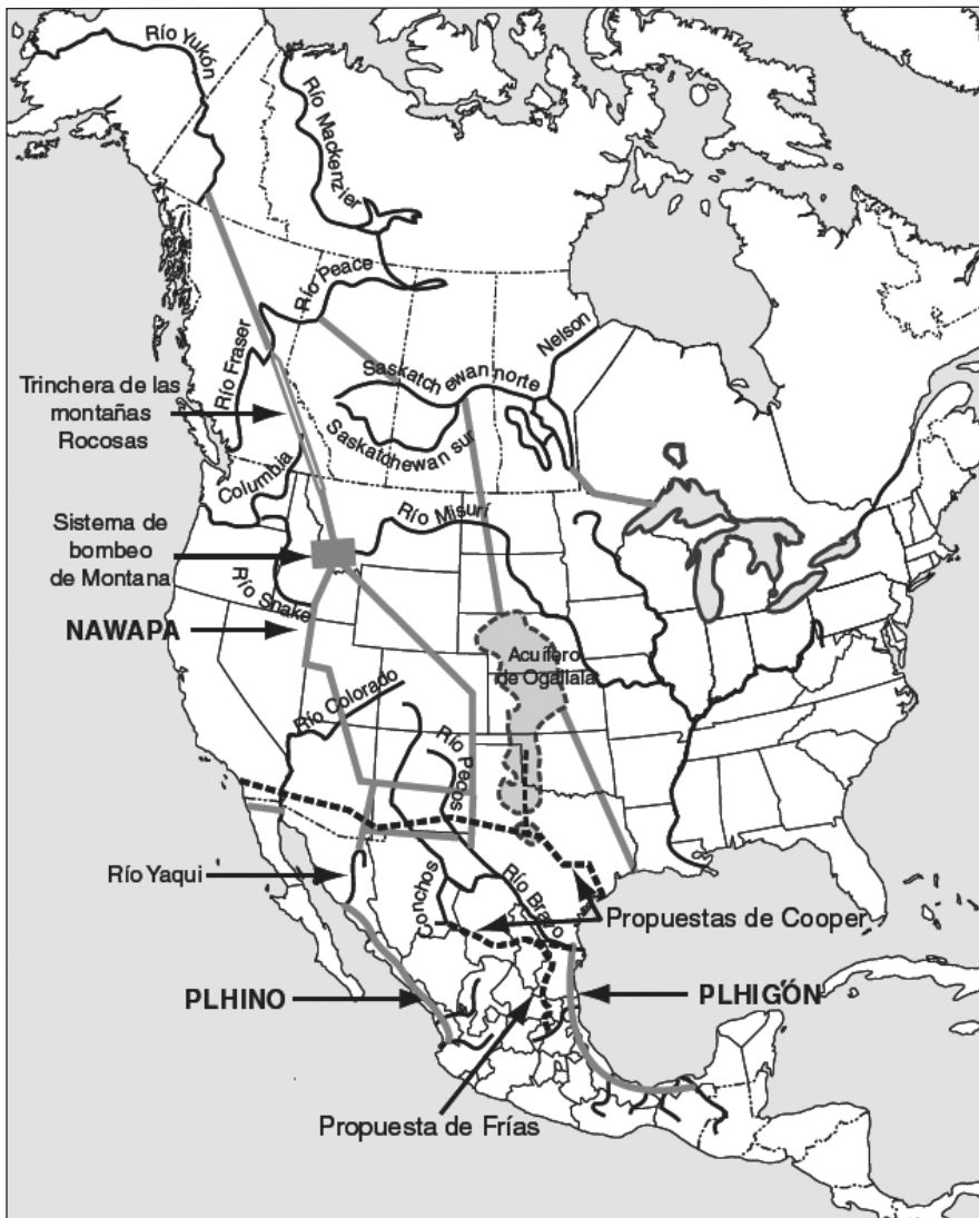
Figura 1 Norteamérica: 'NAWAPA-Más'
